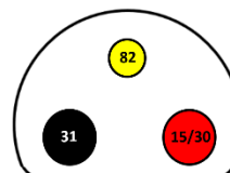
Ansicht Stecker
