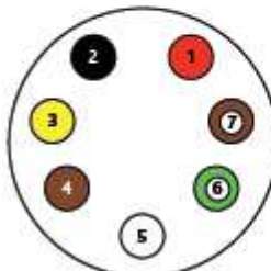
Ansicht Stecker
