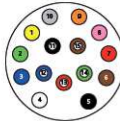
Ansicht Stecker
