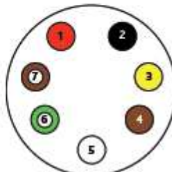
Ansicht Kabelseitig
