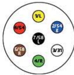
Ansicht Kabelseitig
