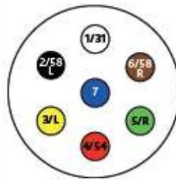
Ansicht Stecker
